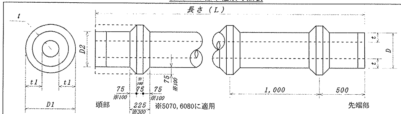
節くいの標準種別寸法表
