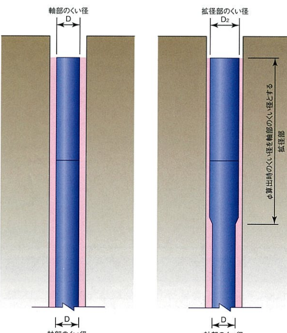
① 拡径部無しの場合 ② 拡径部有りの場合
