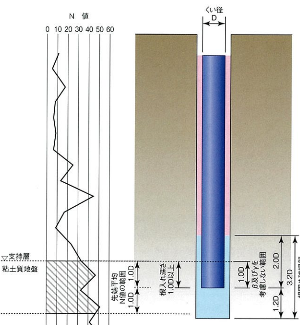
くい先端適用範囲
